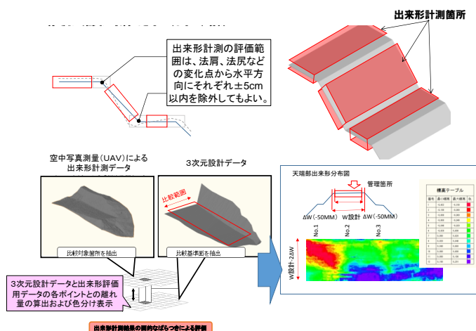
図 1-17 出来形管理図表 作成の流れ
