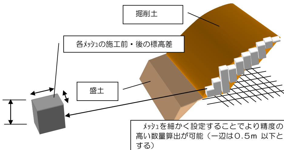
図 1-20 点高法による数量算出の条件と適用イメージ
