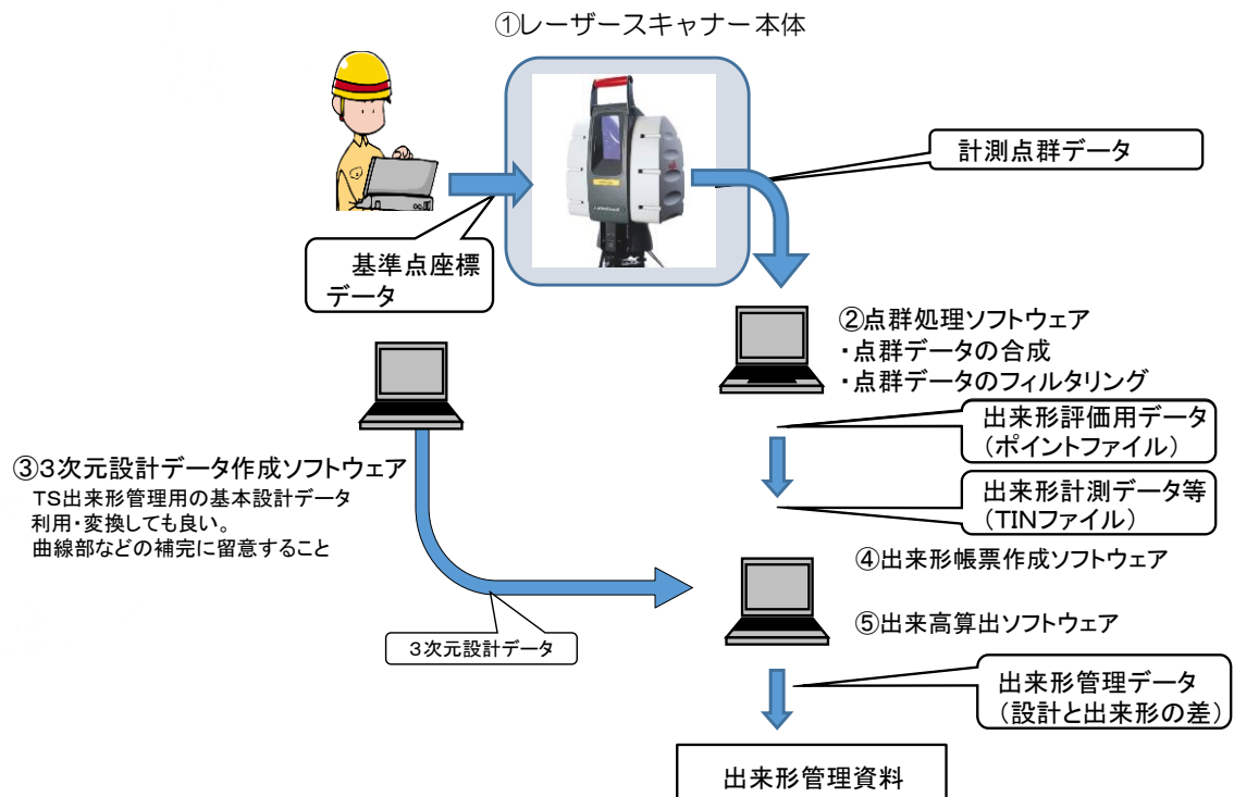
図 1-5 LSによる出来形管理機器の構成例
