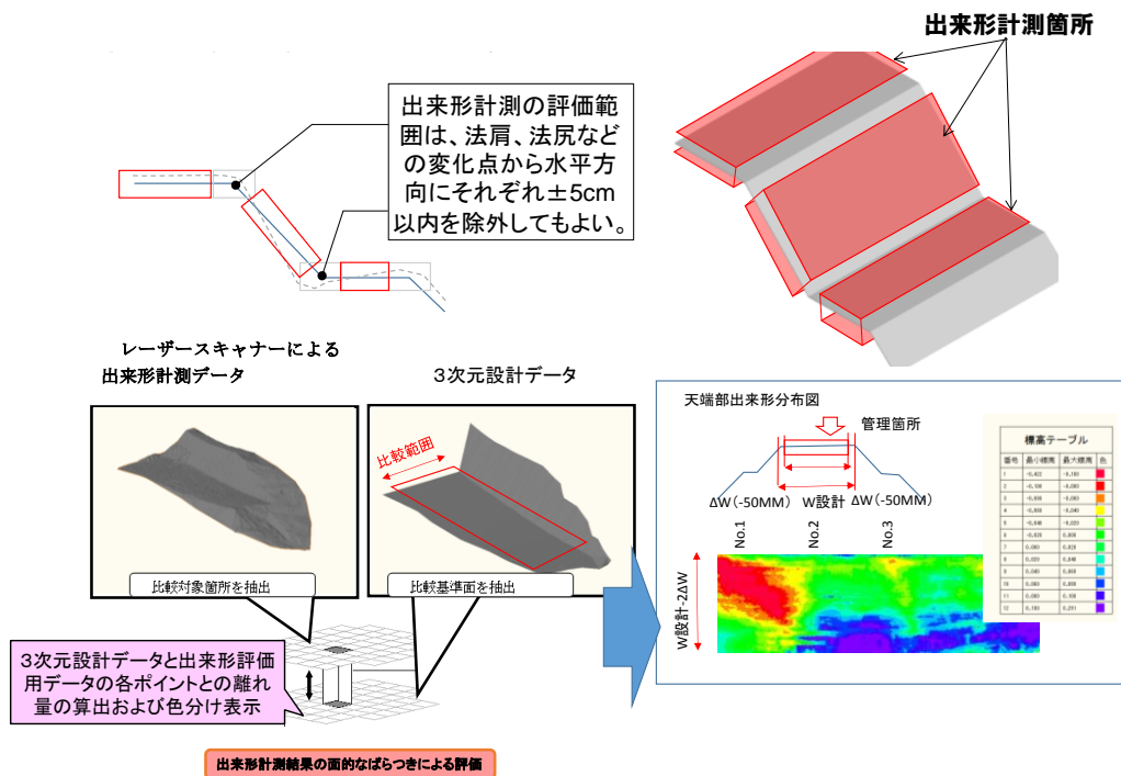
図 1-12 面的な出来形管理分布図のイメージ
