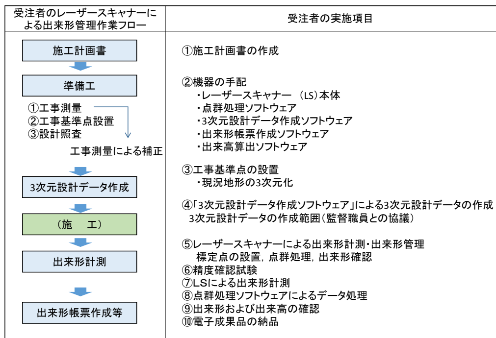
図 1-1 LSによる計測の手順
