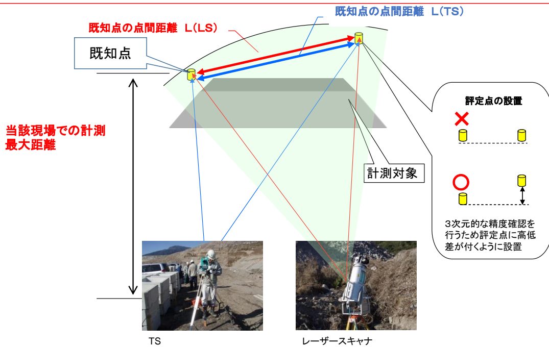
図 4-1 精度確認試験の配置イメージ図
