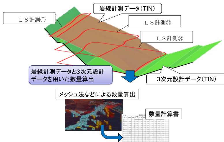
図 1-14 設計変更(岩区分)のための数量算出イメージ
