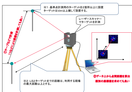
図 4-2 LSと既知点の設置
