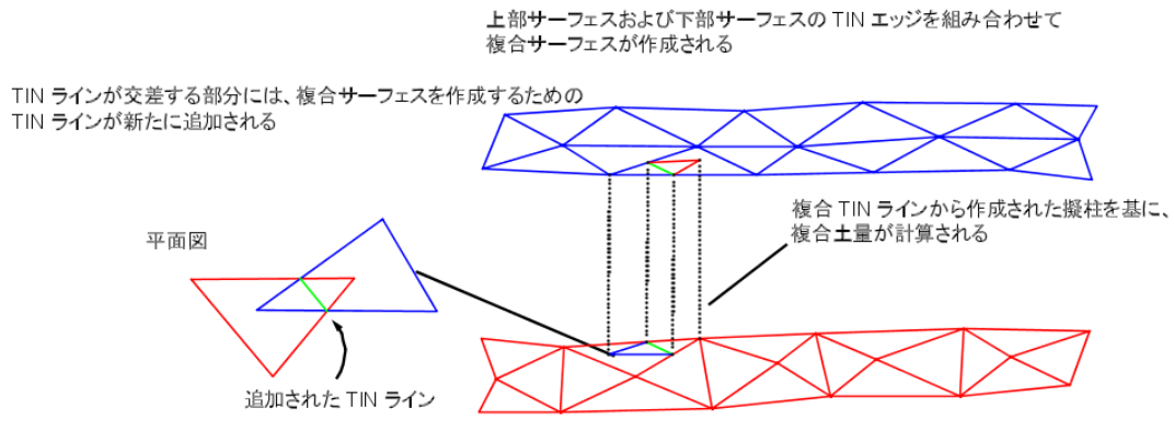
図 1-23 プリズモイダル法による数量算出
