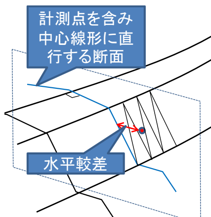
図 1-11 水平較差の算出ロジックのイメージ
