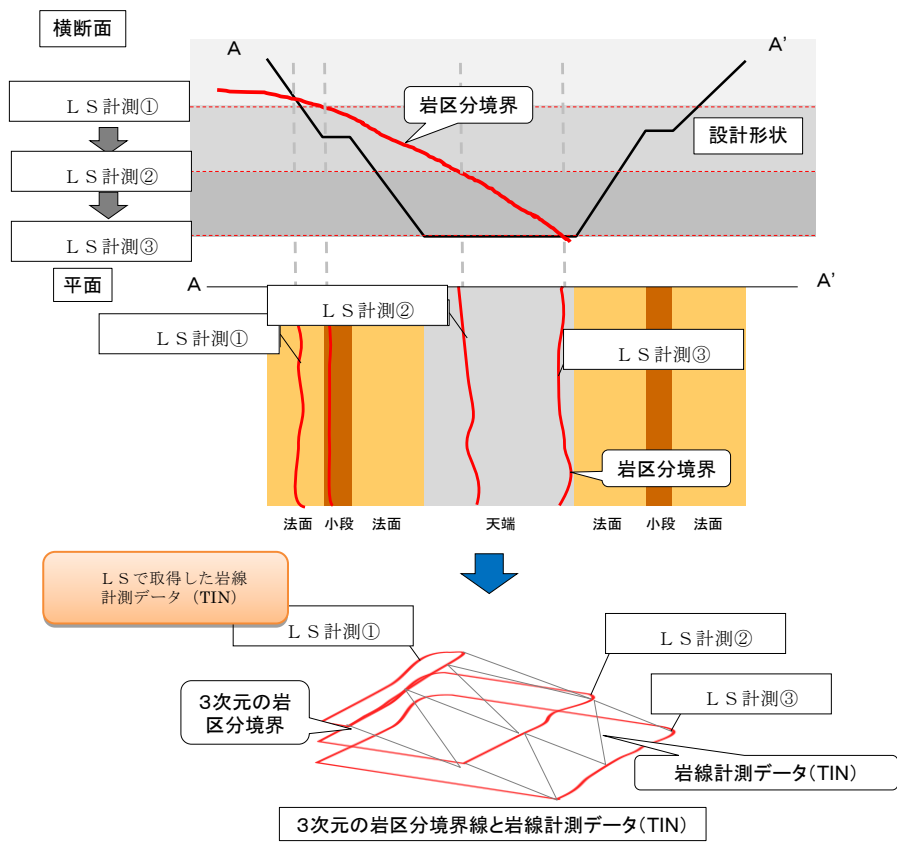
図 1-15 LSで取得する岩区分境界のイメージ
