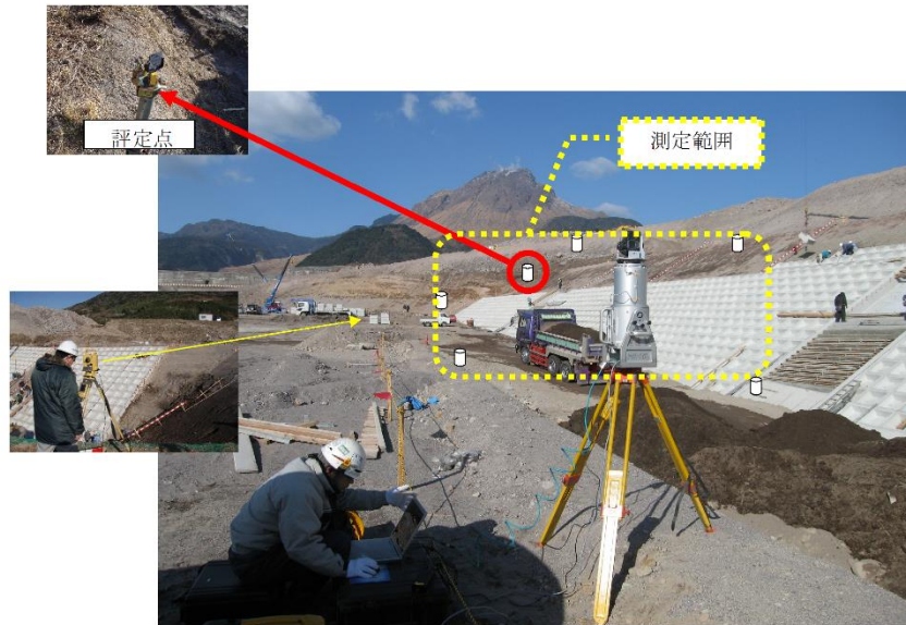
図 1-16 LSと標定点の配置（例）
