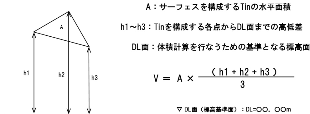
図 1-2 2 TIN分割等を用いた求積による数量算出
