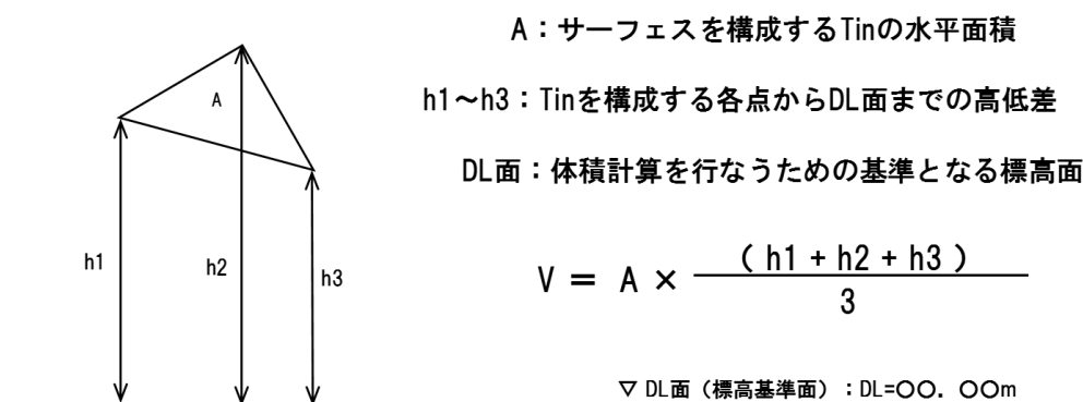
図 1-20 TIN分割等を用いた求積による数量算出
