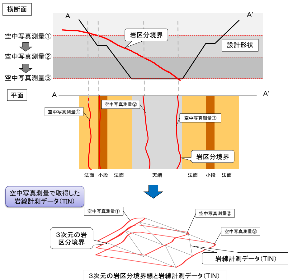
図 1-14 空中写真測量で取得する岩区分境界のイメージ
