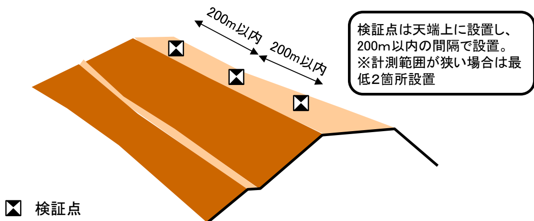
図 4-1 精度確認試験の配置イメージ図
