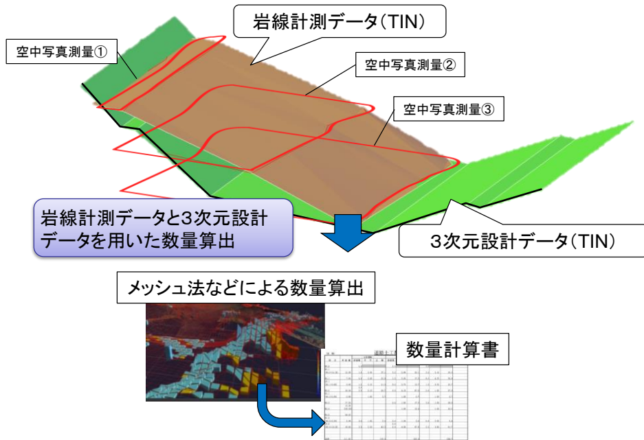
図 1-13 設計変更（岩区分）のための数量算出イメージ
