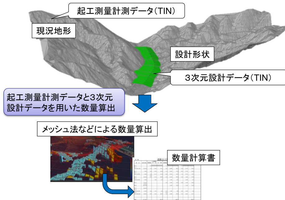
図 1-12 設計照査のための数量算出イメージ
