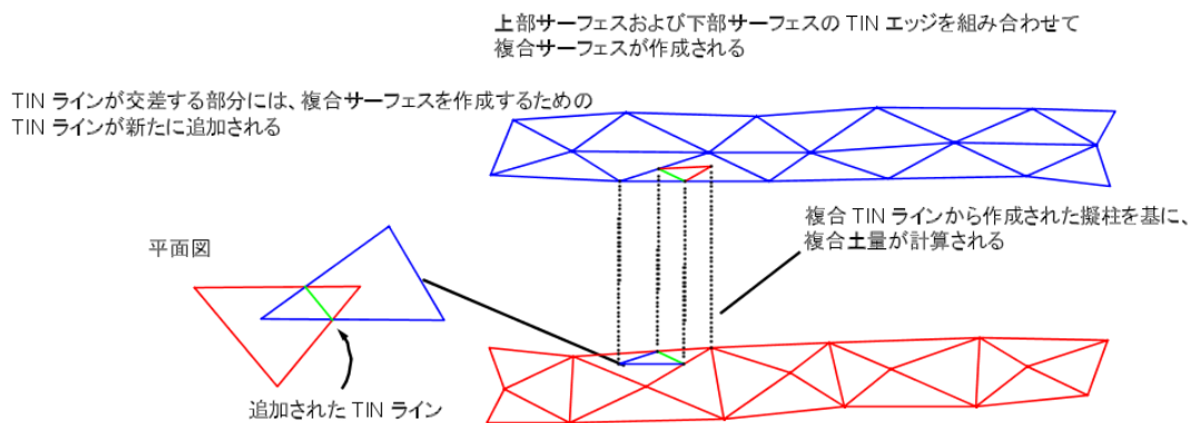
図 1-21 プリズモイダル法による数量算出
