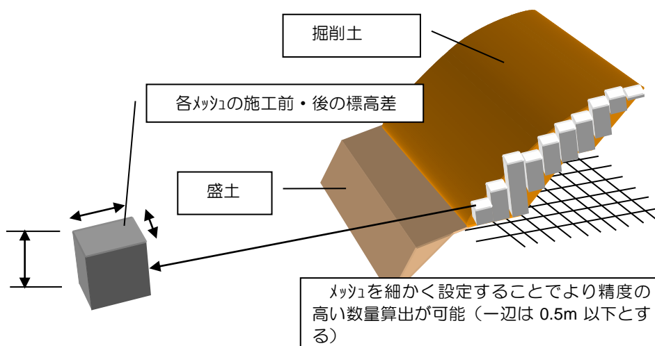
図 1-18 点高法による数量算出の条件と適用イメージ
