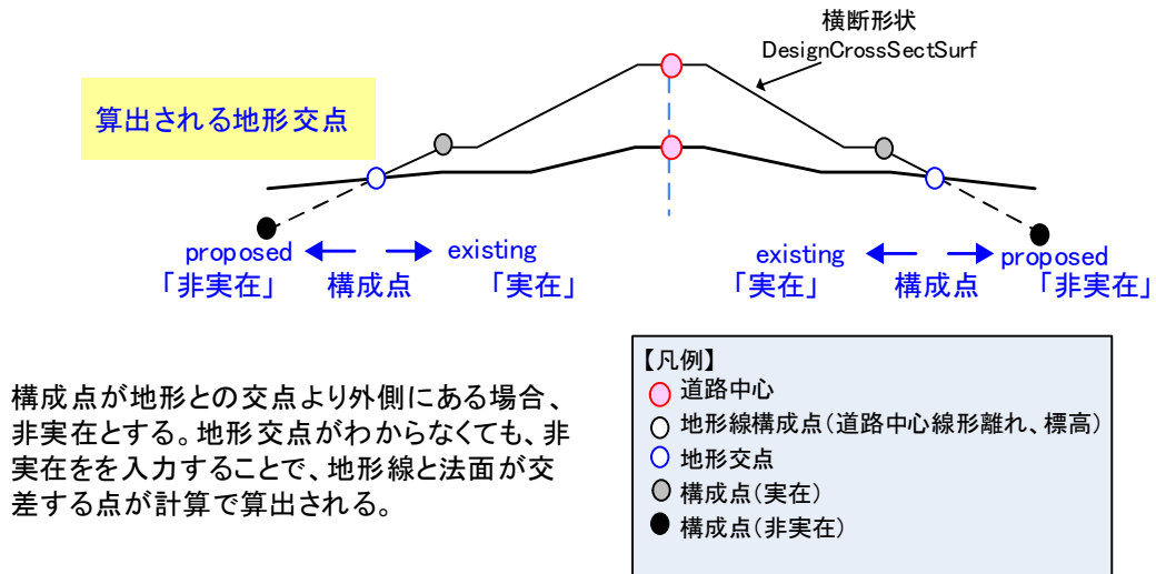
図 13 地形とのすり付けイメージ
