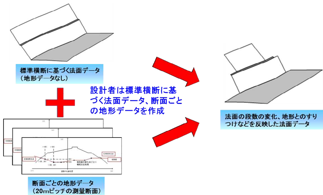
図 12 法面・地形のデータ作成
