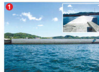
工事名 長崎地区広域漁港整備工事(内防波堤(E)改良) 施工者 西海・田浦JV 技術者 山田 聡 工事内容 防波堤を撤去・新設する工事です。
