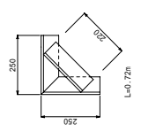
プラケット詳細図 S=1:10
