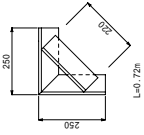
ブ ラ ク エ ッ ト 詳 細 図 S=1:10
