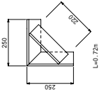
フラケット詳細図 S=1:10
