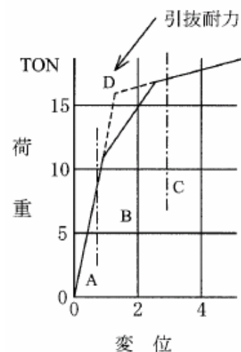
図 4-1 ロックボルト引抜試験
