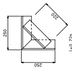
プラケット詳細図 S=1:10
