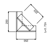
ブラケット詳細図 S=1:10
