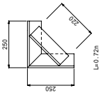
ブラスケット詳細図 S=1:10
